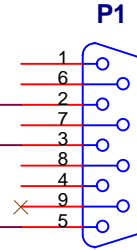
CONNECTEUR DB9 MALE
