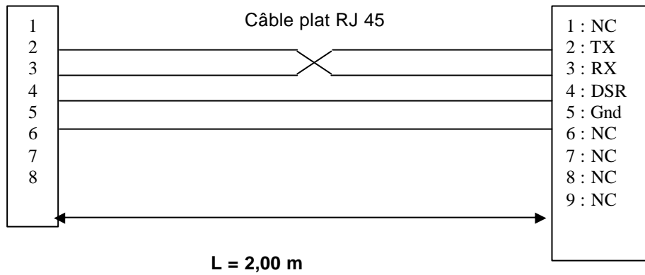
Connecteur RJ45
