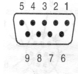
Connecteur RS-232 F
